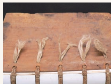
Holzdeckelband nach Bundverlängerung
